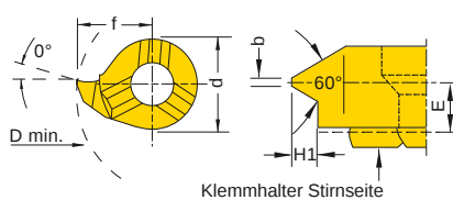
Klemhalter Stirnseite
